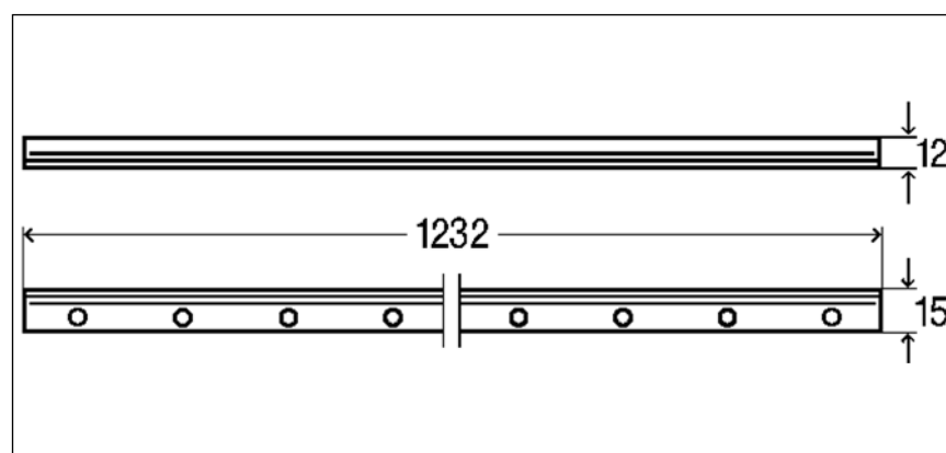
Fig. 2: Dimensions
