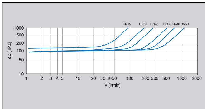
Abb. 3: Leistungsdigramm Druckverlust KRV Press-/Gewindeanschluss
