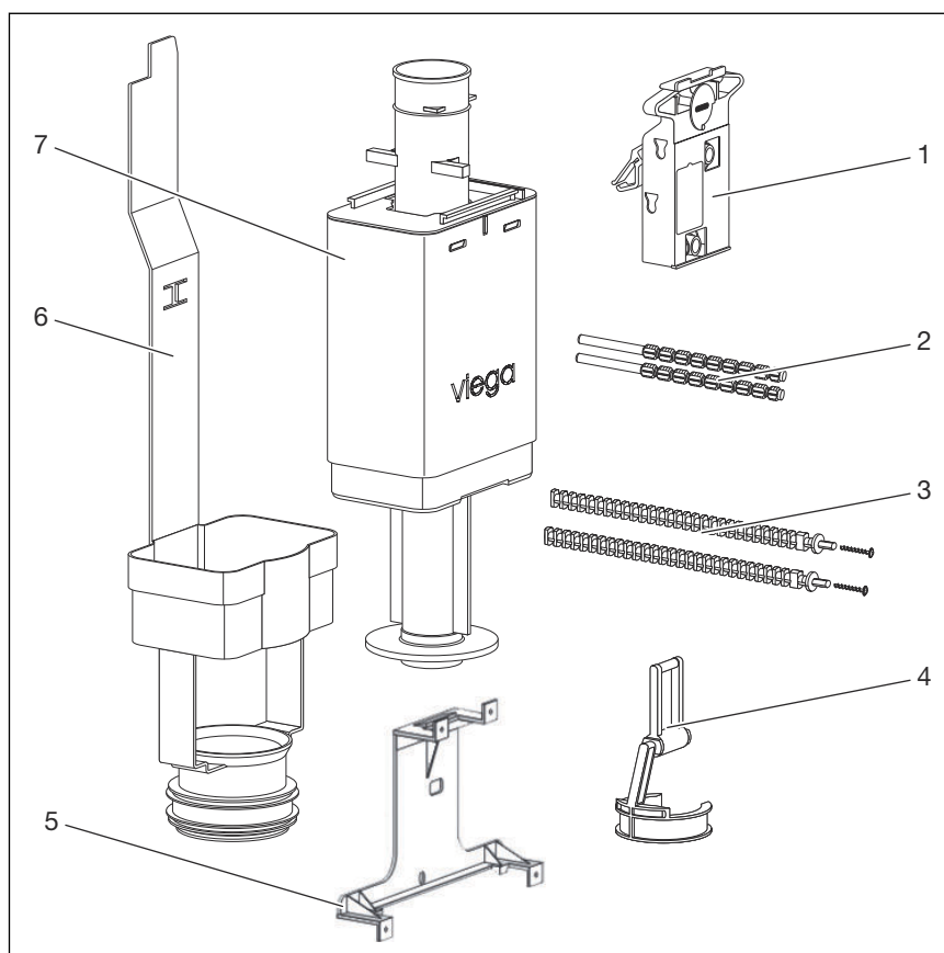
Abb. 1: Ablaufventilset
