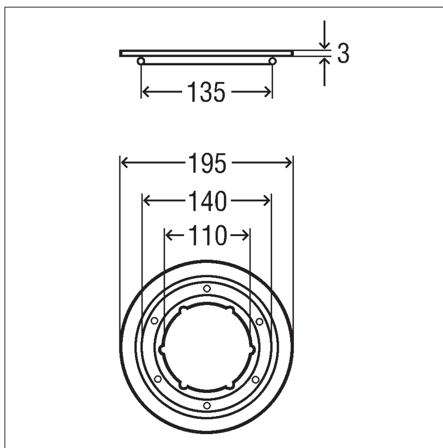
Fig. 2: Disegno dimensionale
