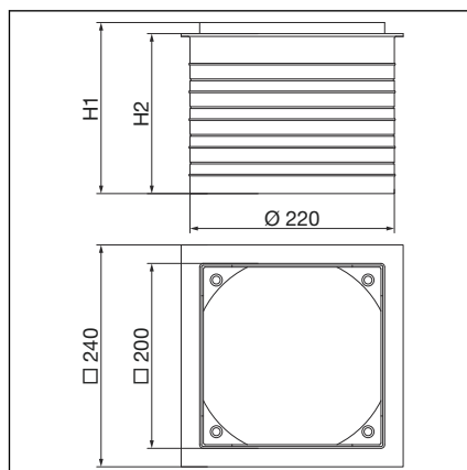
Abb. 1: Einbaumaße
