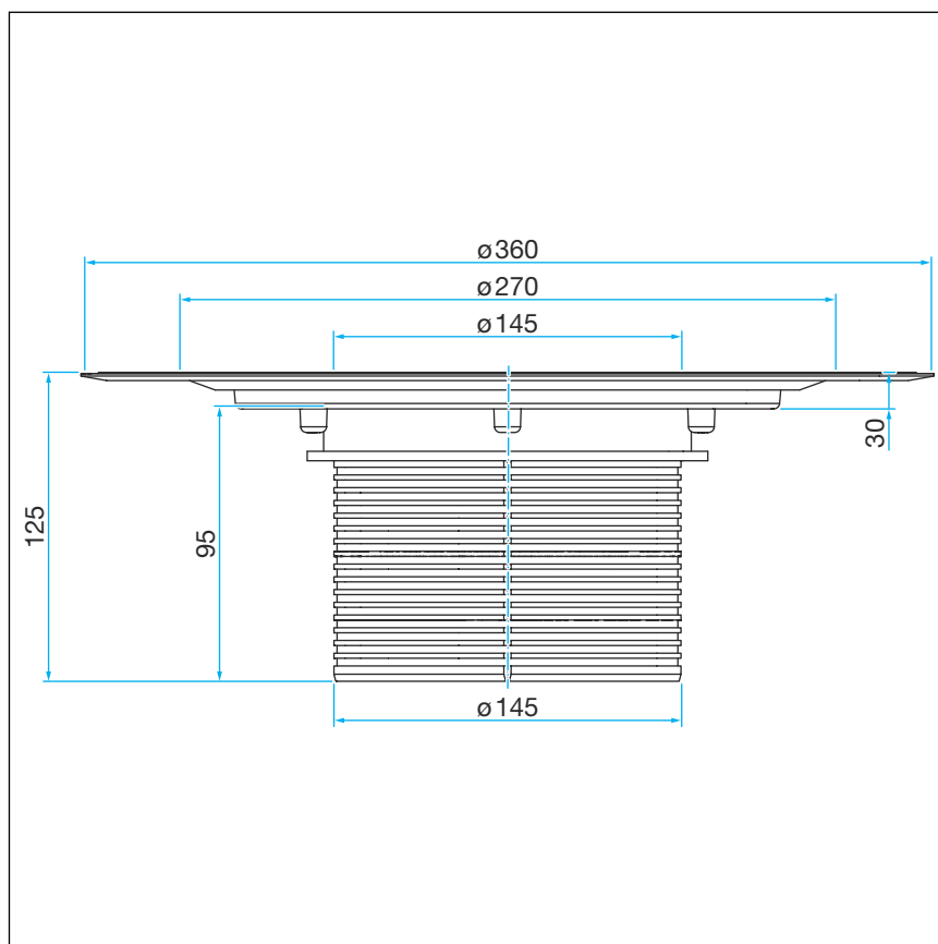
Fig. 3: Disegno dimensionale per modello 4996.1
