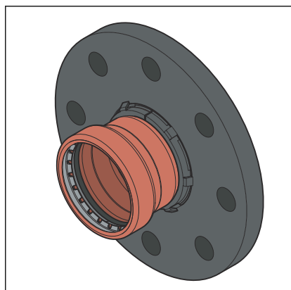
Rys. 7: Kołnierz ruchomy
