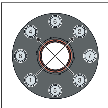
Afb. 8: Profipress G XL zeskant-schroeven kruiselings
