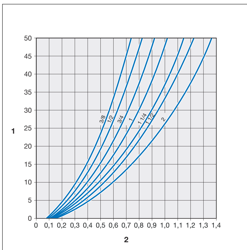
7. ábra: Hajlítás, U-alak, Megapress 3/8-2 col között
