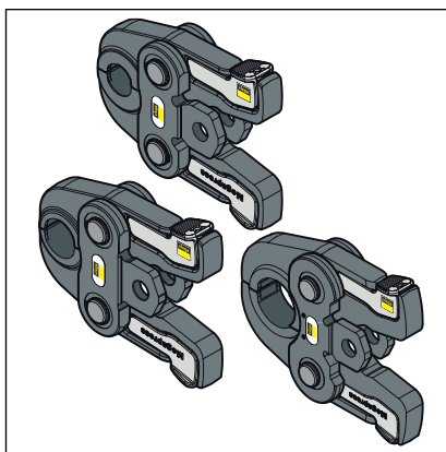
13. ábra: Megapress, prészár
