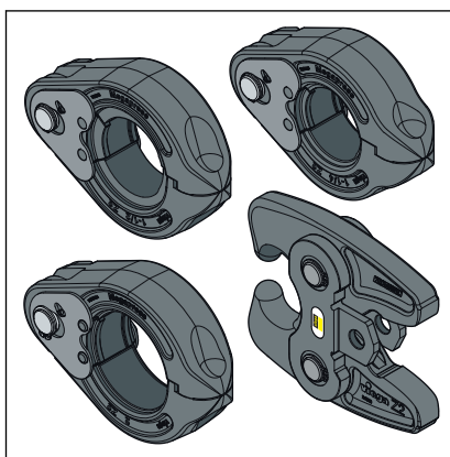
14. ábra: Megapress prészűrűk csuklós behúzópofával
