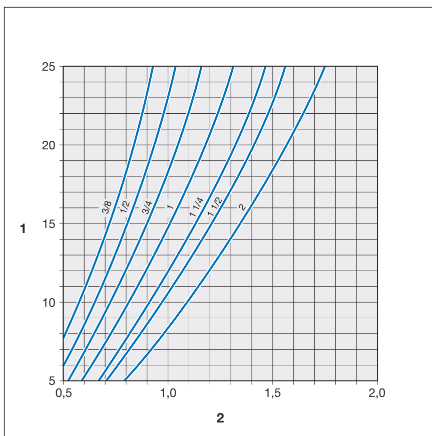
5. ábra: Hajlítás, Z- és T-alak, Megapress 3/8-2 col között
