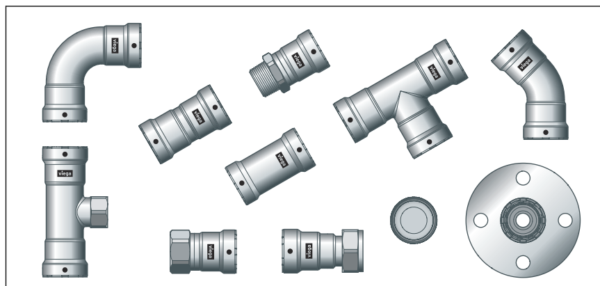
Slika 2: Megapress press spojnice
