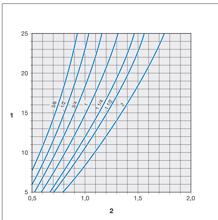
Slika 5: Krakovi savijanja u obliku slova Z i T za Megapress 3/8 do 2 inča
