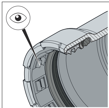
Fig. 15 : Bague crantée
