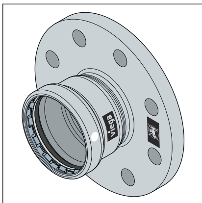
Rys. 16: Kołnierz stały 4259XL / 4259.6XL
