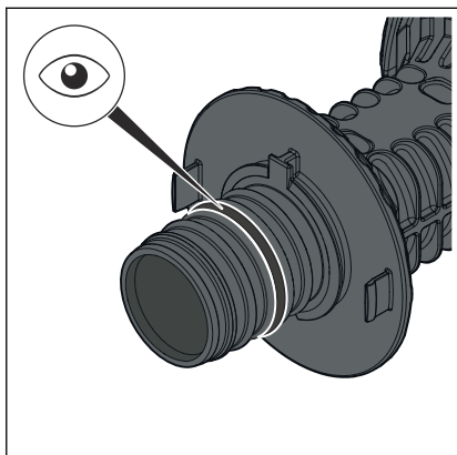
Abb. 3: EPDM-Dichtelement
