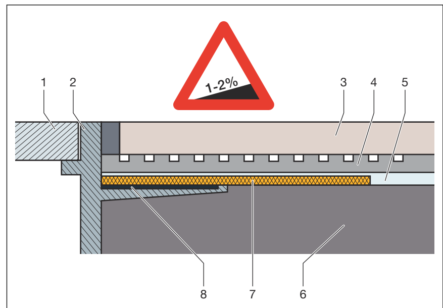
Abb. 10: Aufbauschema der Verbundabdichtung – Estrichgefälle min. 1–2 %
