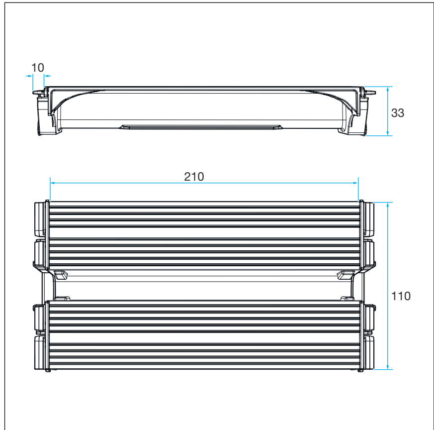
Abb. 14: Abmessungen Verbindungsstück
