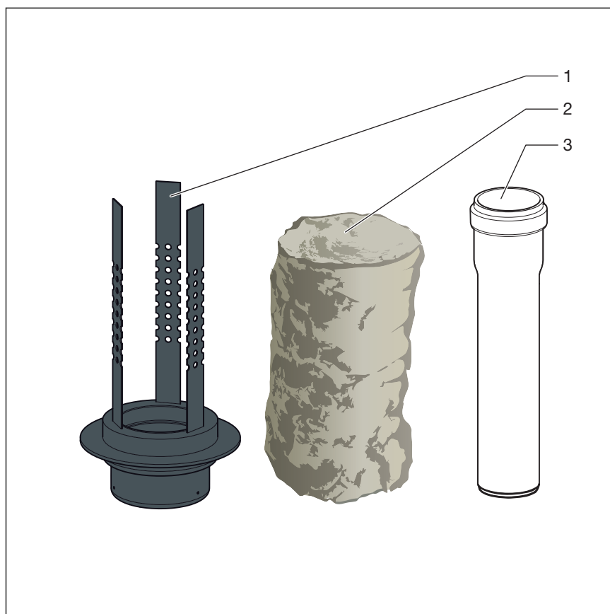
Abb. 1: Brandschutz-Rohrdurchführung
