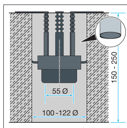
Abb. 2: Maßzeichnung für Modell 4923.5
