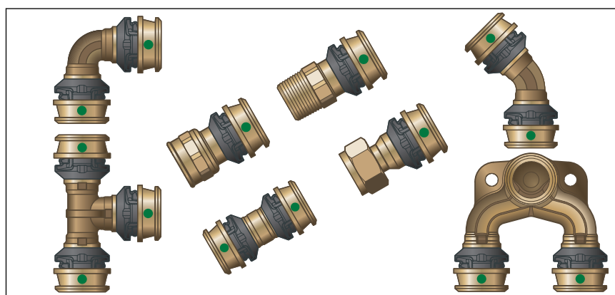
sl. 1: Fitingi za hladno stiskanje Raxofix
