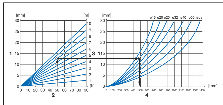
Abb. 2: Raxofix-Mehrschichtverbundrohre (formstabil mit Sauerstoffsperrschicht) – Biegeschenkelänge
